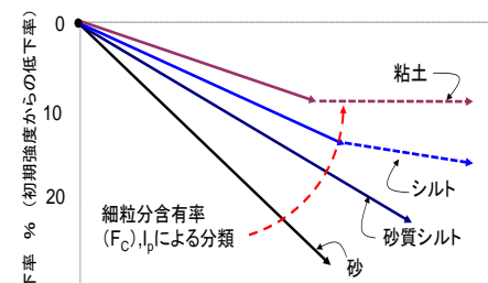
累積ひずみ(両振幅ひずみDA%, 繰返しによって劣化が進む程度)
