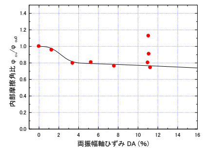
図6 粘性土の標準強度低下曲線
