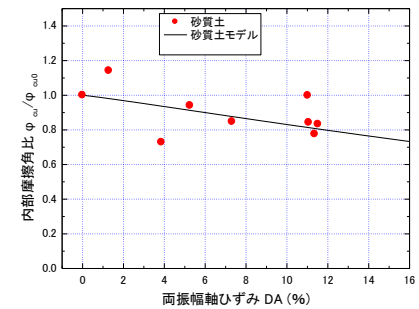
図4 砂質土の標準強度低下曲線
