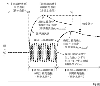
図1 強度低下特性を求める試験方法
