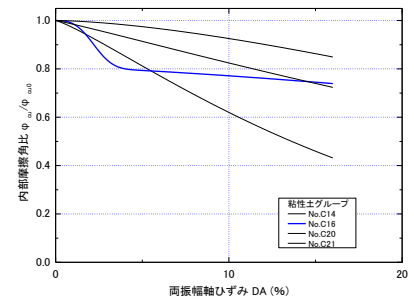
図5 粘性土の強度低下特性
