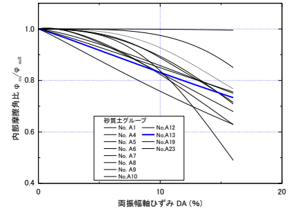
図3 砂質土の強度低下特性
