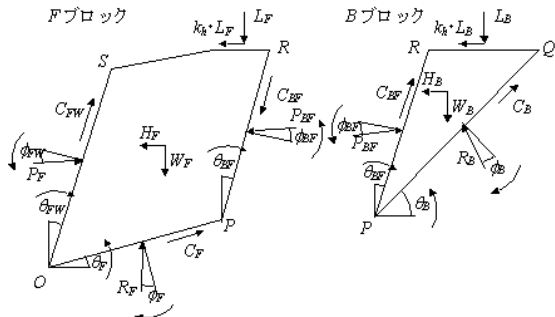
(b)Fブロックの力の釣合い (c)Bブロックの力の釣合い
