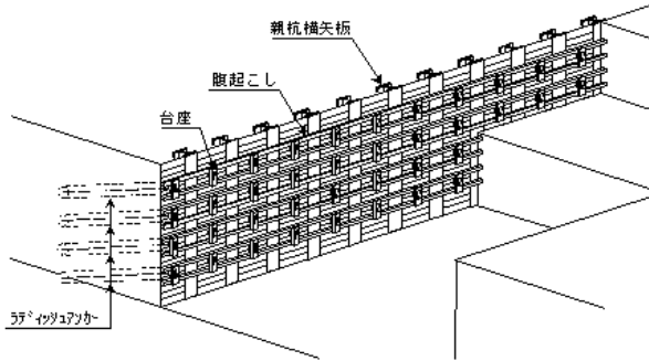
図5 掘削土留工の支保工
