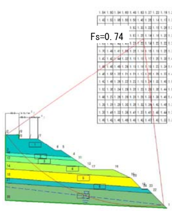
図3 地震時検討断面
