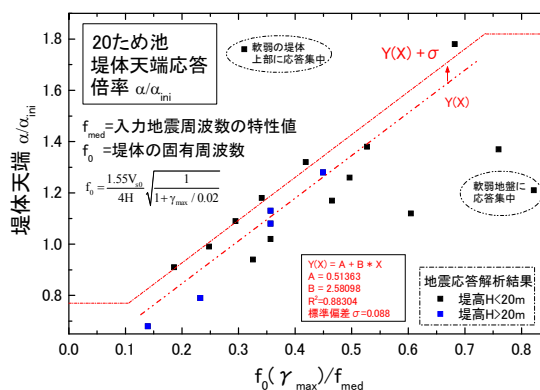
図 2 堤体の応答倍率の簡易推定法
