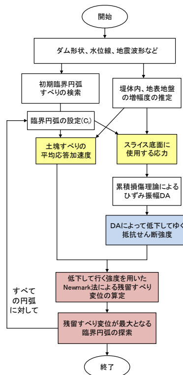
図 1 簡易 NewmarkD 法のフロー
